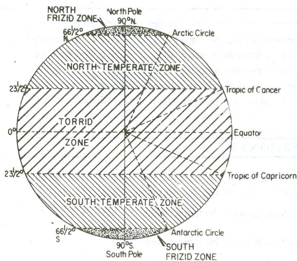
Fig. 13.1 Thermal Zone
