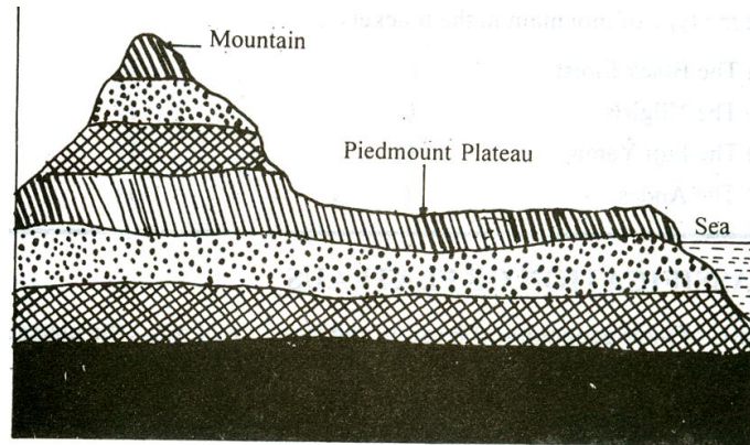
Fig. 7.6 Piedmont Plateau
