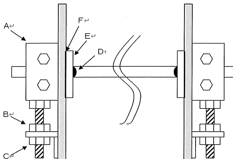
(拡大図)
