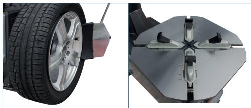
Nářazník s vertikálním a horizontálním nastavením
